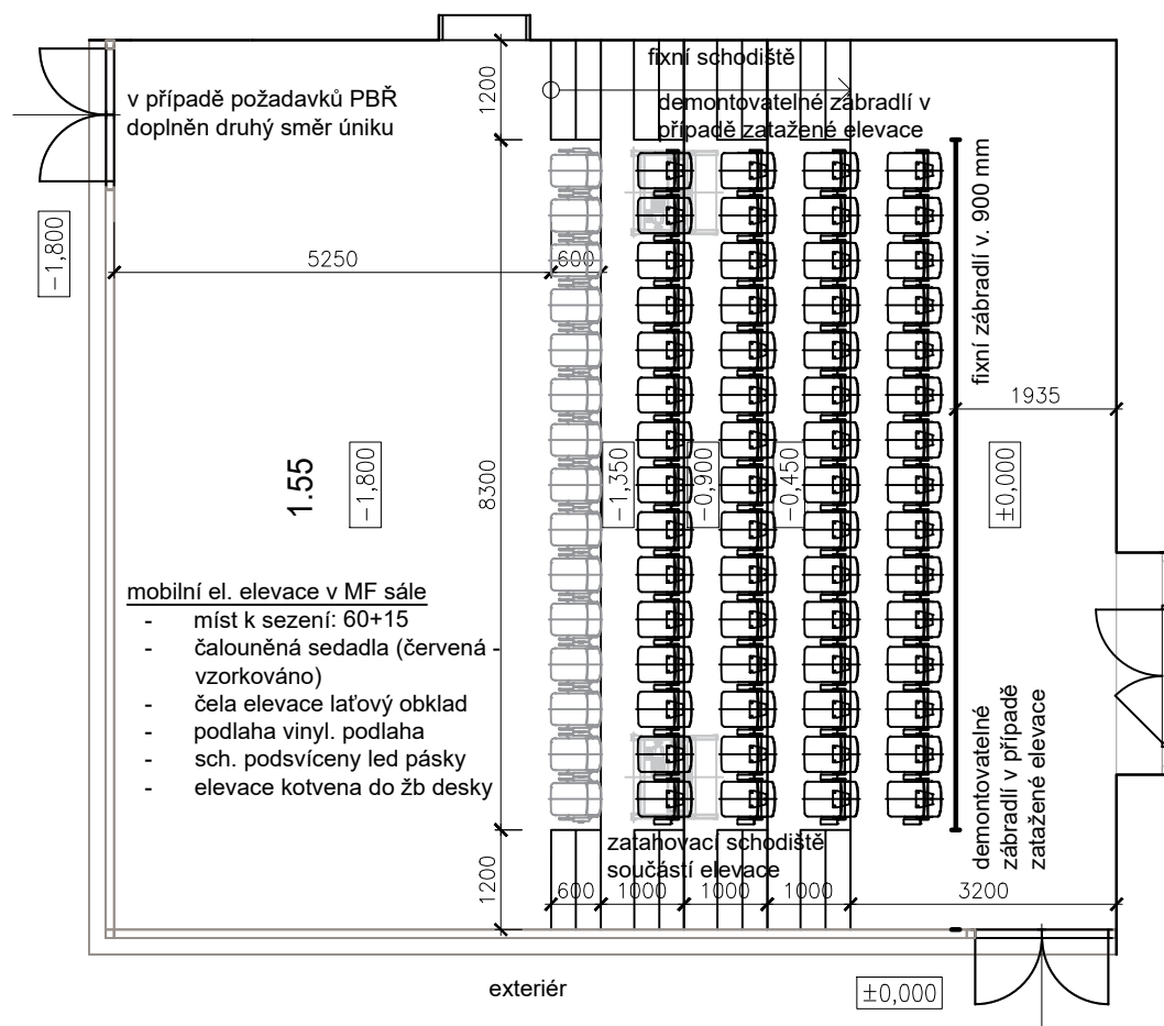
PŮDORYS SÁLU - ROZTAŽENO
