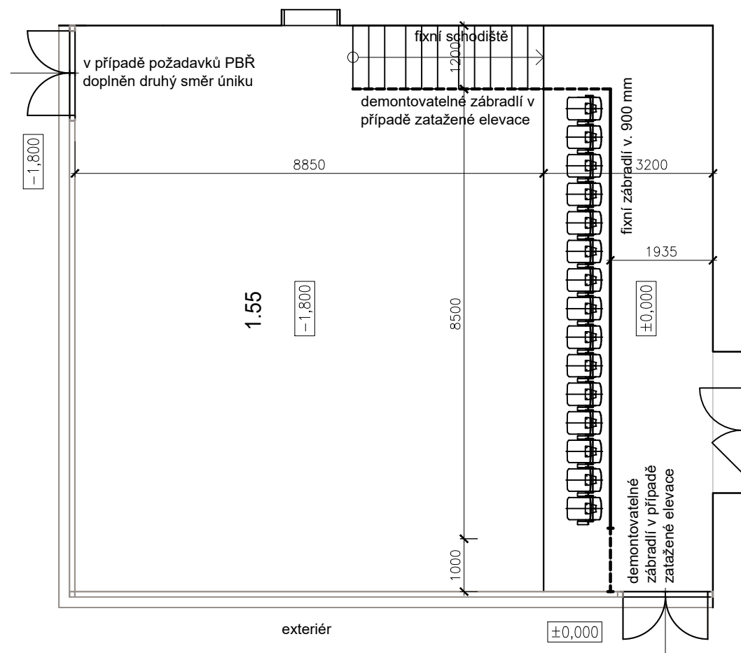
PŮDORYS SÁLU - SLOŽENO
